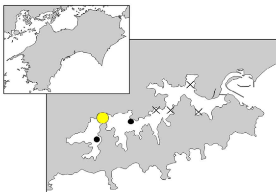
アレキサンドリウム属
